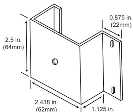
1940-L Garage Door Bracket
